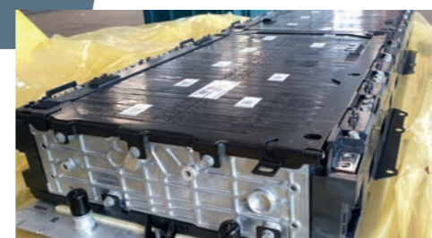
Komplette Hochvoltbatterie wird für die Montage vorbereitet.
